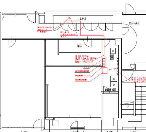
庁舎 6 階機器配置図
